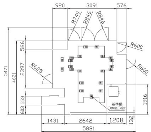
上蓋圖 Top View
