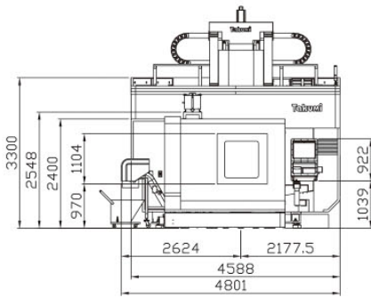
側視圖 Side View
