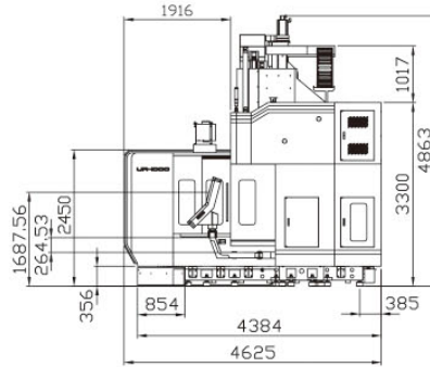
正視圖 Front View
